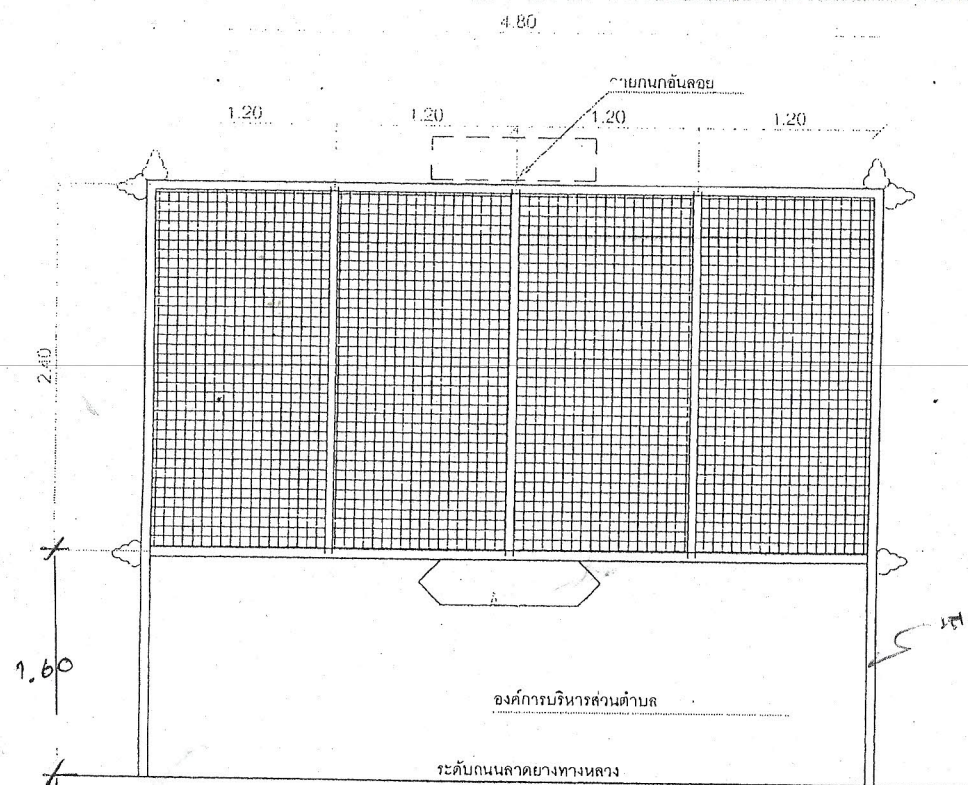
แบบด้านหน้า ฐานราก 1:50
