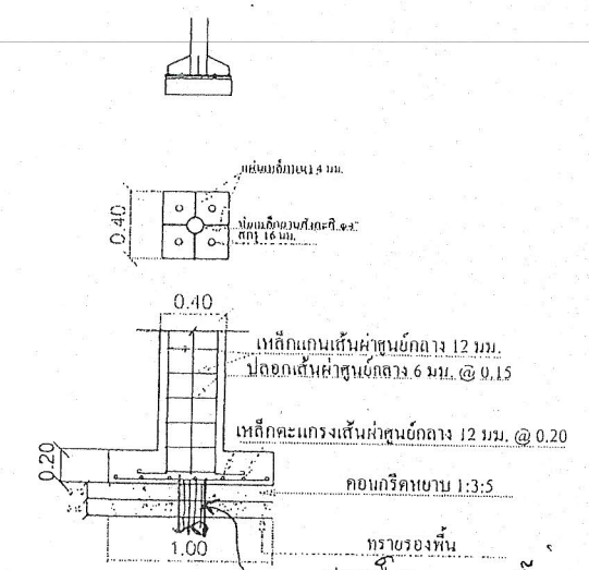
แบบขยาย ฐานราก 1:20 ทรายรองพื้น ๓ ชั้น ขนาด ๑๕ ซม. ๗ ชั้น ขนาด ๖.๐ ซม.
